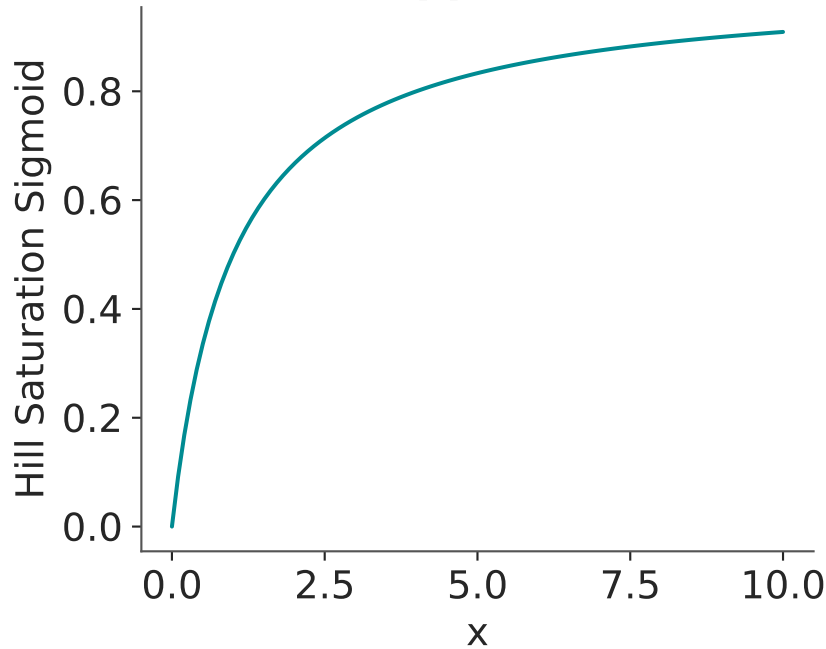
Kappa = 1
