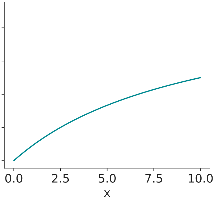
Kappa = 10
