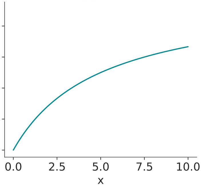
Kappa = 5
